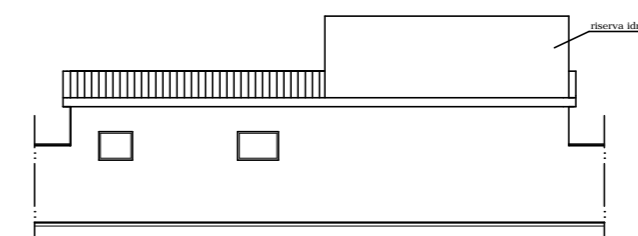
PROSPETTO C
