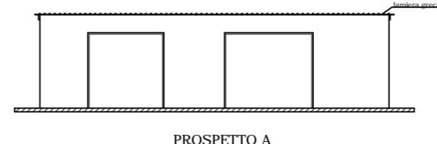
PROSPETTO A
