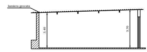
SEZIONE A-A
