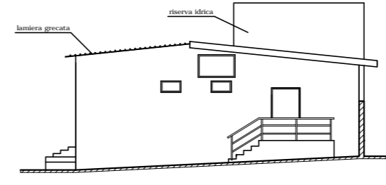
PROSPETTO B
